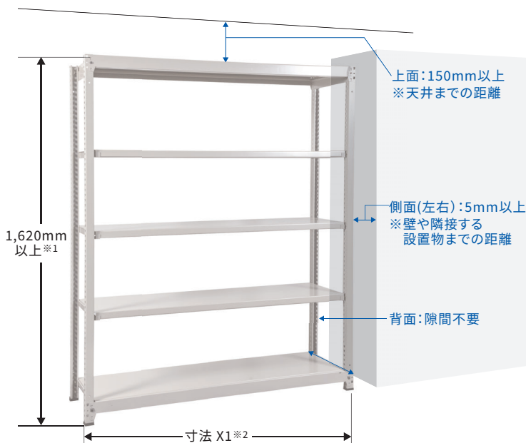
本体側面寸法図
