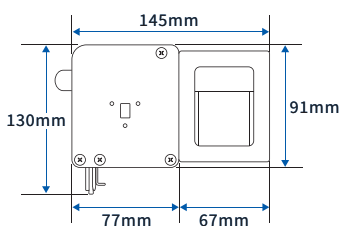
本体側面寸法図
