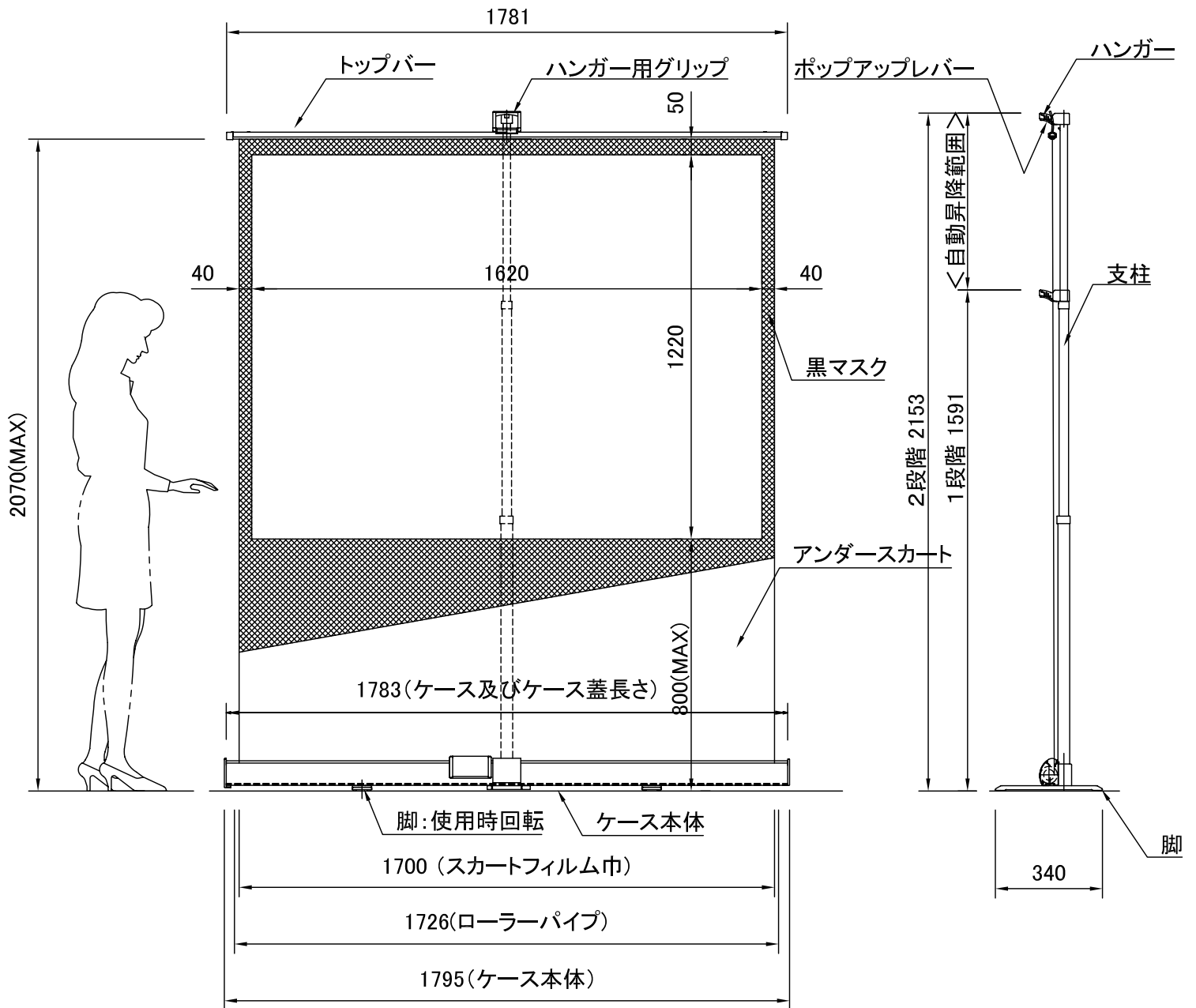
スクリーン設置図 S=1/20
