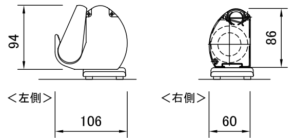
スクリーン収納時ケース外寸 S=1/6
