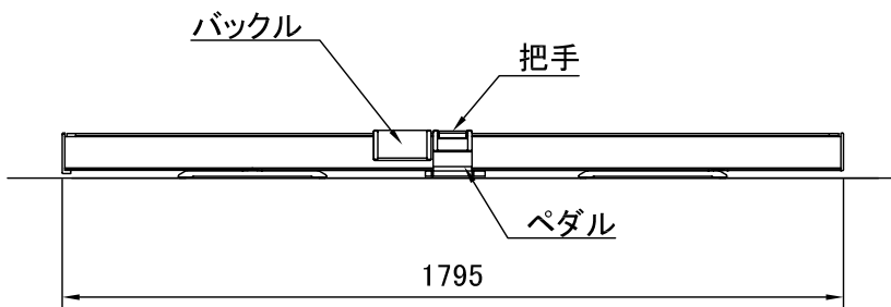
スクリーン収納時ケース外寸 S=1/20
