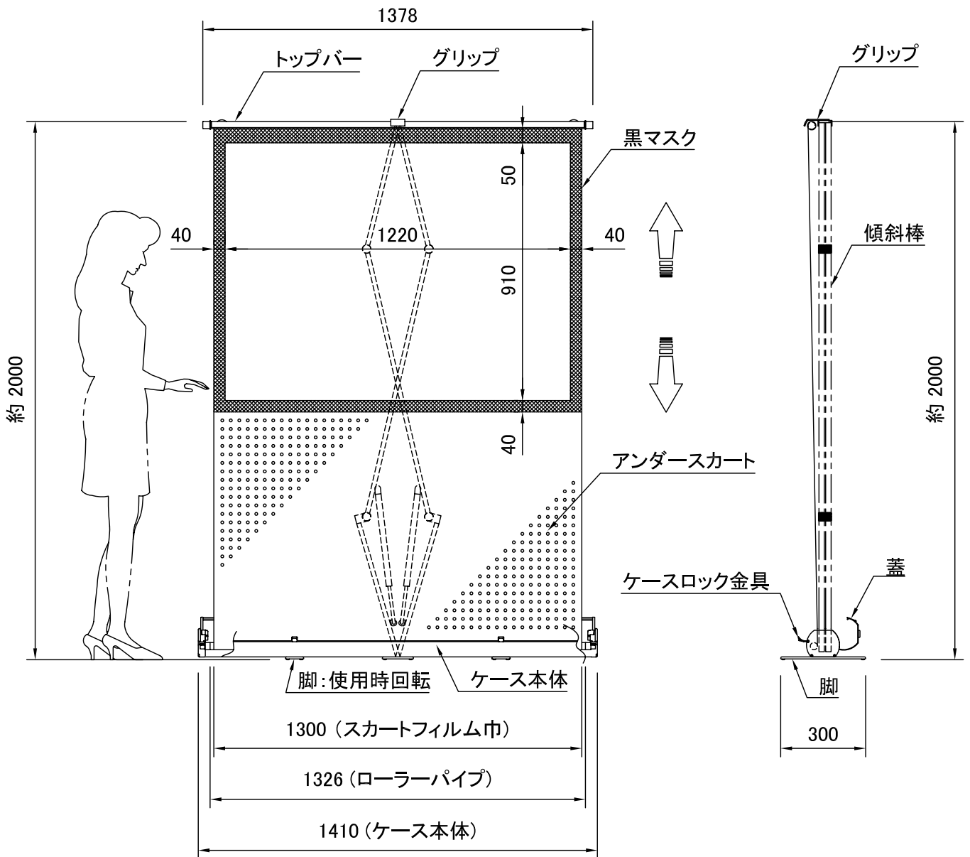
スクリーン設置図 S=1/20
