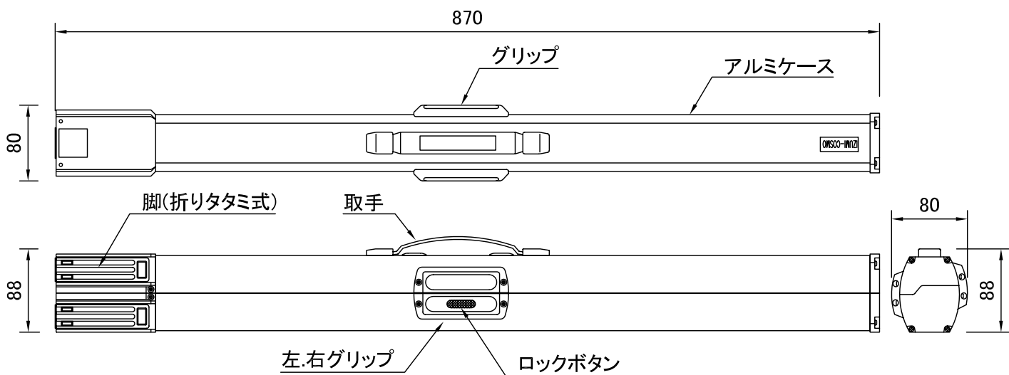
スクリーン収納時ケース外寸 S=1/6
