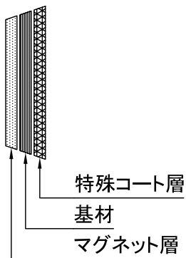
WOLスクリーン構造図
